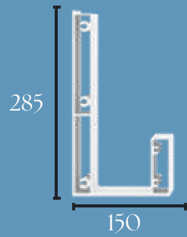
Poutre intégrée Integrated Beam
